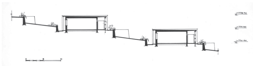
ד"א ברוצקוס, תכנית וחתך של ביתני המעבדות, גבעת רם, 1955 (עיזבון ברוצקוס)
